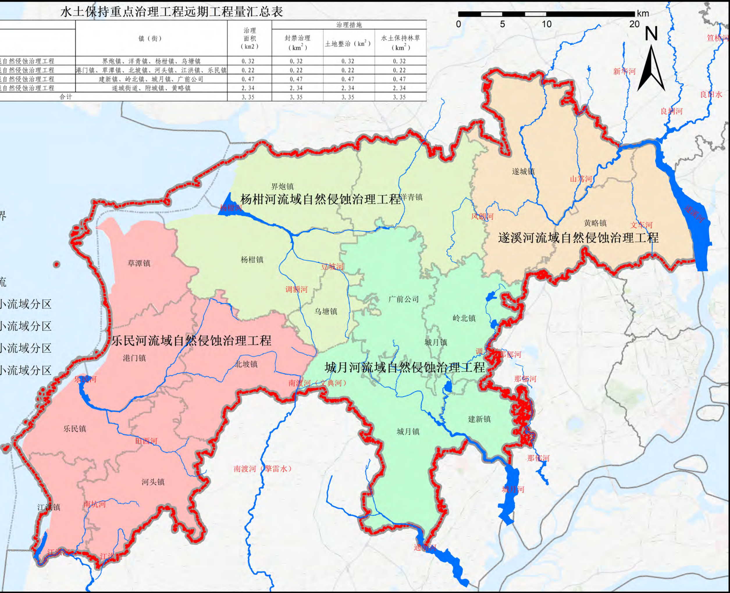
附图14 遂溪县远期重点综合治理工程分布图
