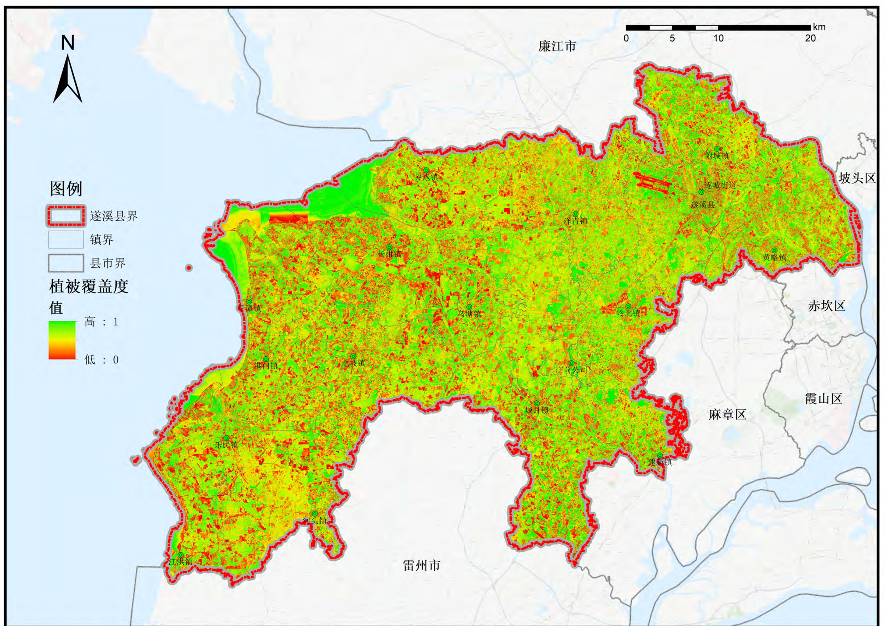
附图05 遂溪县植被覆盖度分布图
