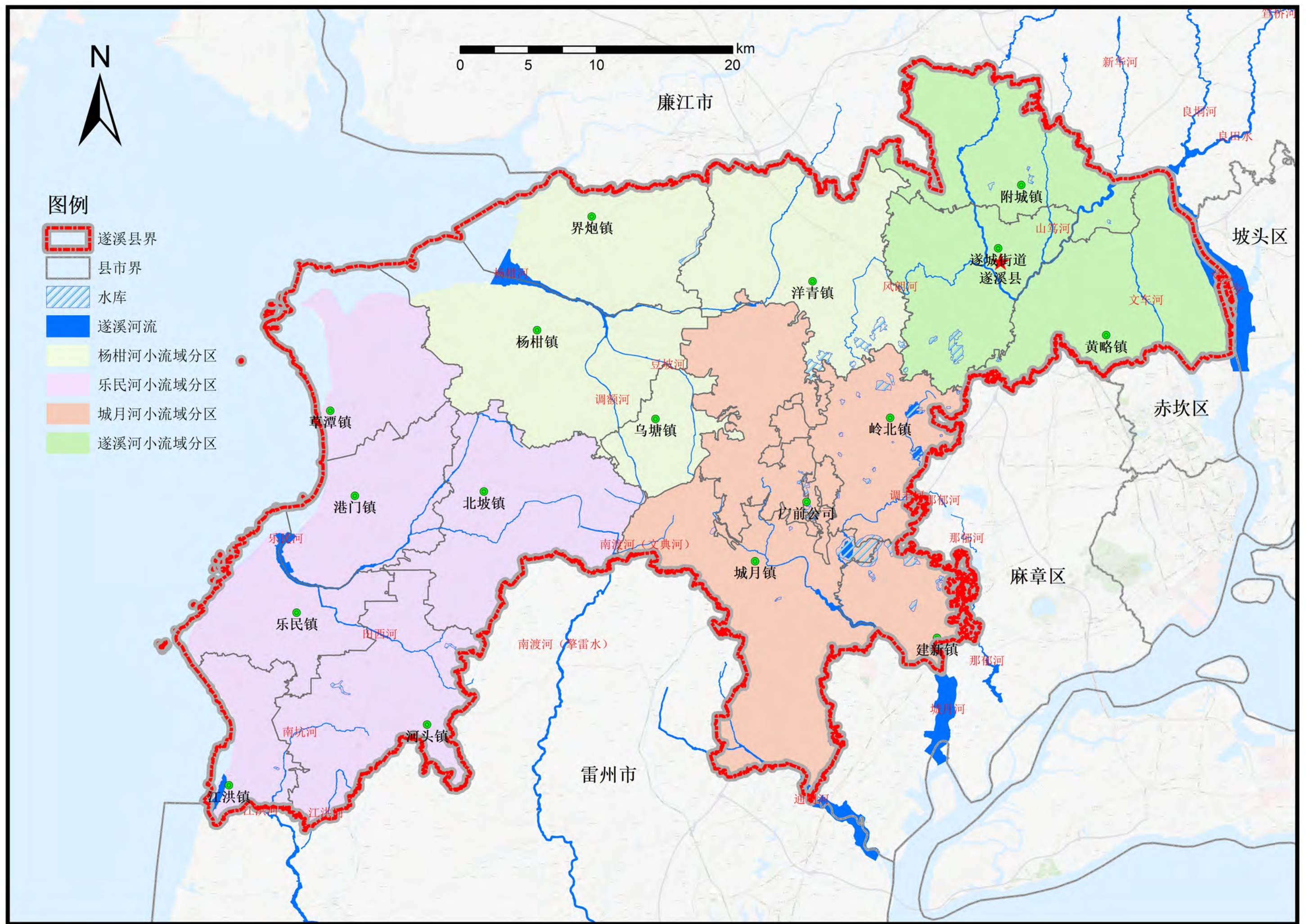
附图02 遂溪县水系图
