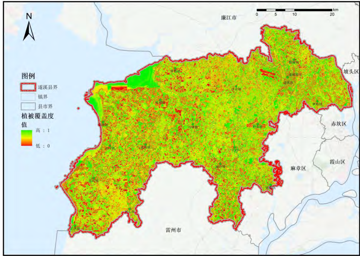
图 1-4 遂溪县植被覆盖度分布图
