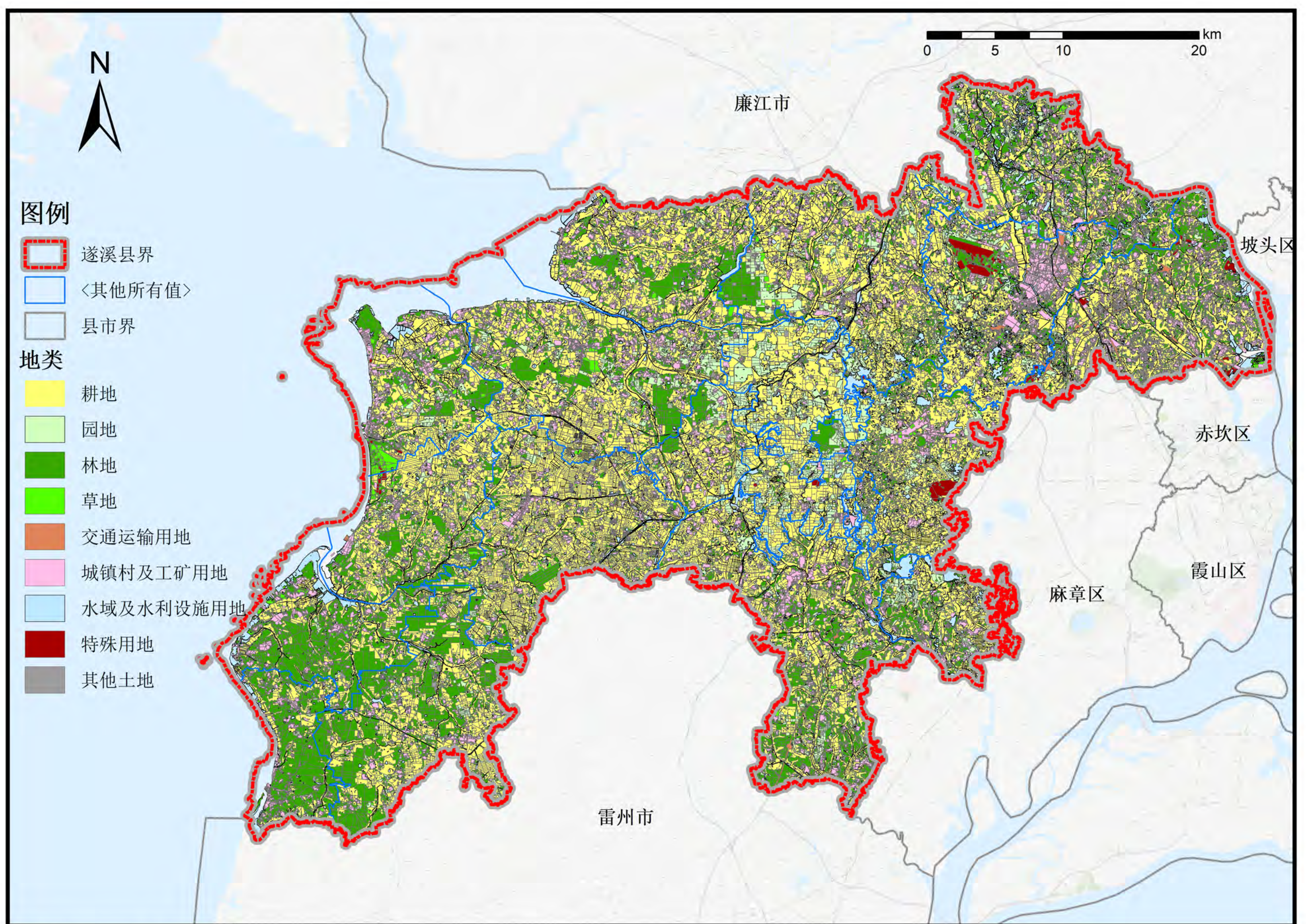
附图06 遂溪县耕地、园地、林地分布图
