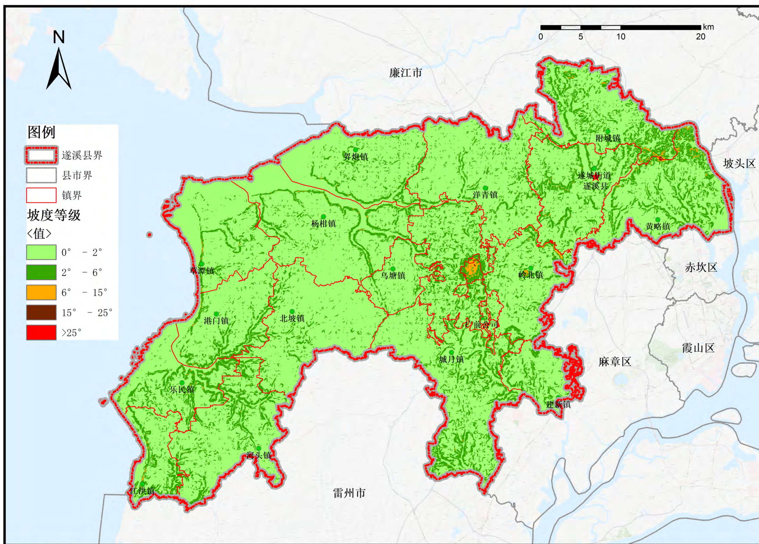
附图04 遂溪县坡度等级分布图
